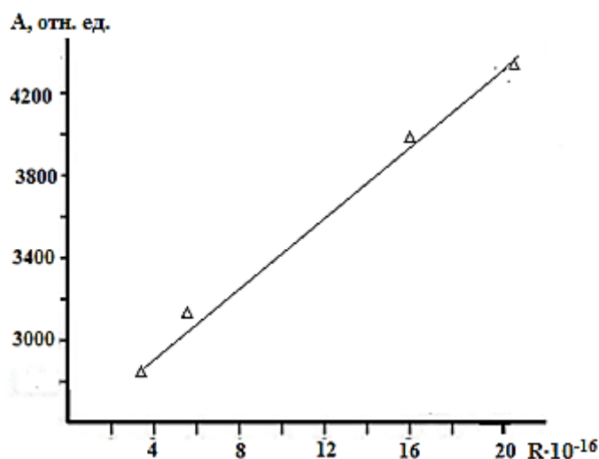
Рис.4.6. Зависимость интегральной интенсивности гидроксилных групп от количества присоединившихся спин-меток.
