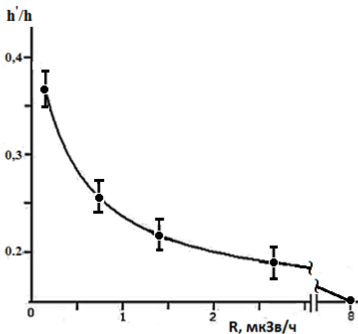
Рис.4.8. Зависимость параметра h'/h от радиационного фона места произрастания листьев репейника.
