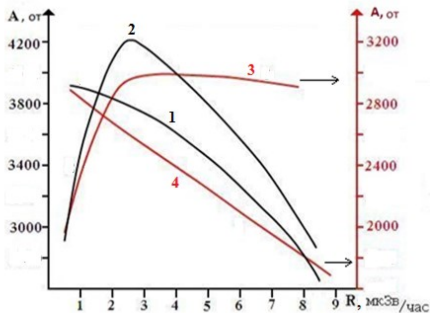
Рис.3.3 Зависимость относительной интегральной интенсивности полос поглощения от уровня радиации: 1-листья до КО , 3–листья после КО; 2– корневища до КО, 4– корневища после КО.
