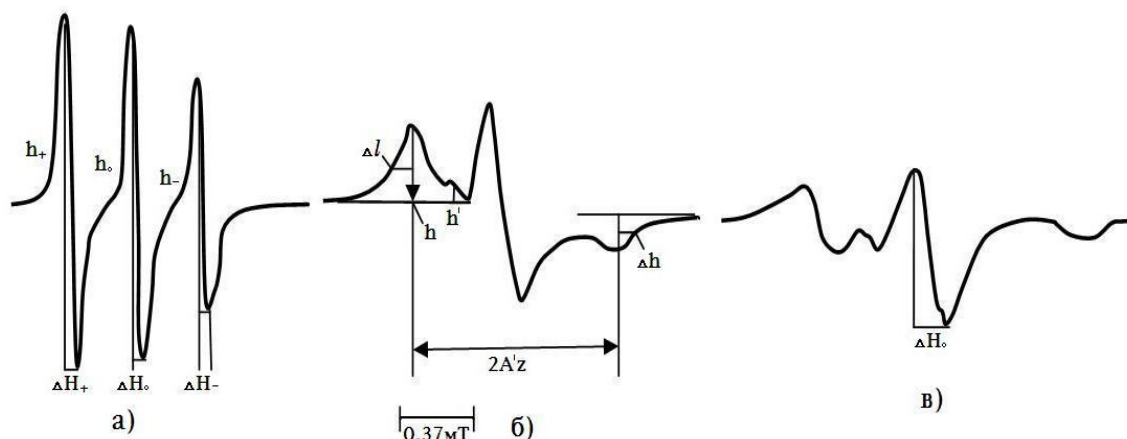
Рис. 4.12. ЭПР-спектры нитроксильного свободного радикала (I): а- в этаноловом растворе с концентрацией 4 \cdot 10^{-3} М/л; б-в исходных листьях ПЛ; в-в обработанных пестицидами листьях ПЛ.
