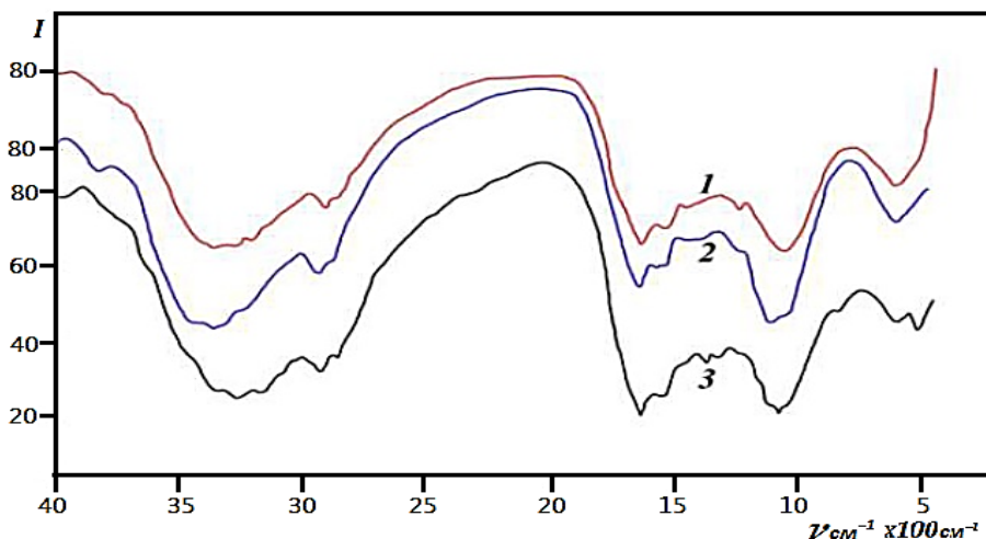
Рис. 3.9. ИК-спектры листьев донника после КО, собранных в: 1–Худжанде, 2– «Дигмае» и 3–Гулистане.
