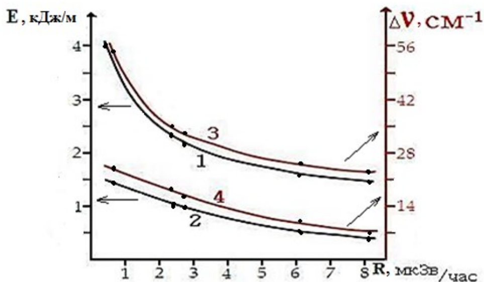
Рис.3.4. Зависимость энергии межмолекулярного взаимодействия и смещения частоты полосы поглощения \Delta\nu(\text{cm}^{-1}) в репейнике от уровня радиации: 1, 3 – листья; 2, 4 – корень.
